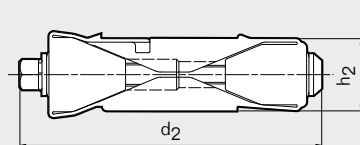
Uncompressed 没有压缩的 / Enspannt / Descomprimido / Desserré
