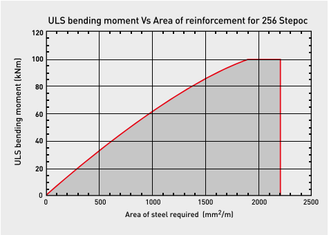
256mm STEPOC
