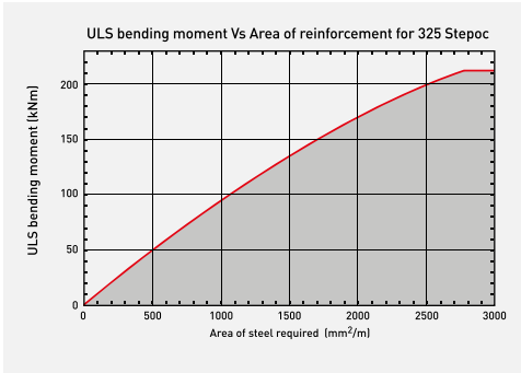
325mm STEPOC
