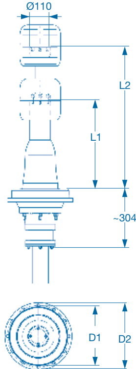
Transformer KTEV
