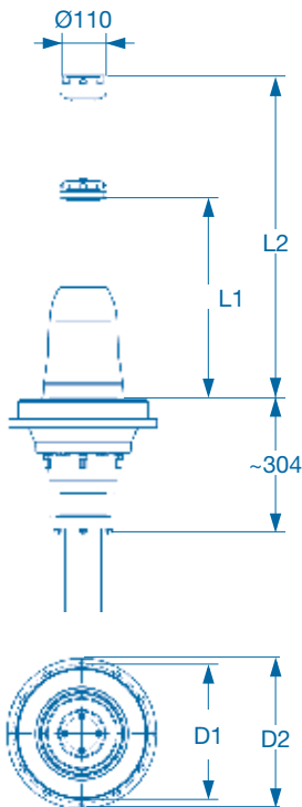
GIS KSEV
