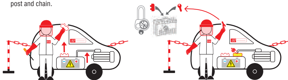
3) Lock in «OFF position»
