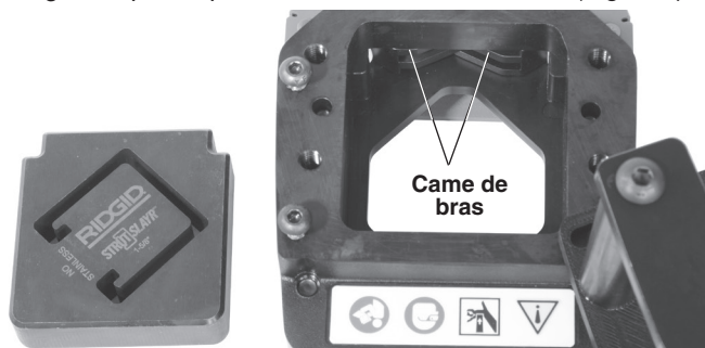
Figure 4 – Lubrification de la cisaille de chemins de câble
