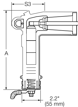
M.O.V.E. Arrester
